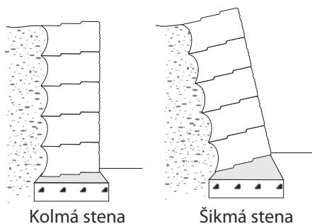
Spôsob uloženia - blok lúpaný
