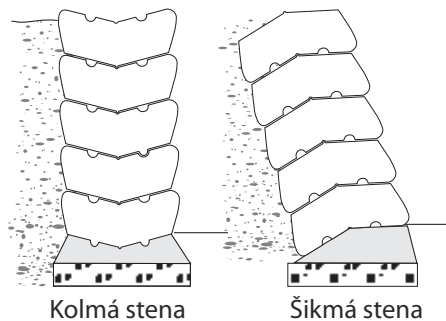
Spôsob uloženia - blok svahový kaskáda
